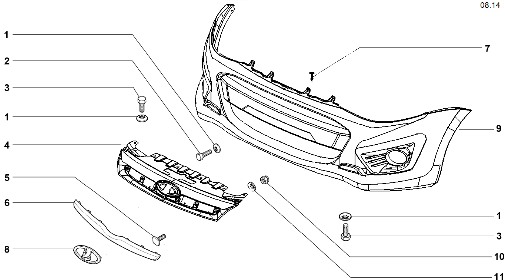
БАМПЕР ПЕРЕДНИЙ
